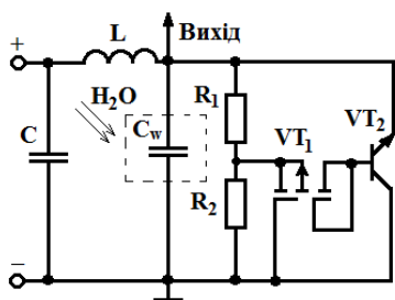
Рисунок 1. Електрична схема частотного перетворювача вологості
