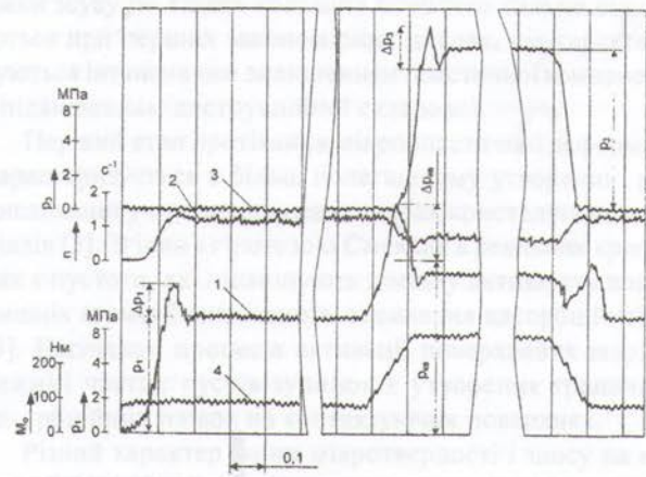
Рис. 6. Осцилограма перехідних процесів вмонтованого гідравлічного приводу конвеєра, чутливого до навантаження, за тиску відкриття p_{zv}=12 МПа, крутильної жорсткості c_p=0,37 \cdot 10^{-3} Н·м/рад; f_3/f_4=0,6 : 1 — зміна тиску в напірній гідромагістралі першого гідромотора; 2 — зміна частоти обертання виконавчої ланки приводу; 3 — зміна тиску в напірній гідромагістралі другого гідромотора; 4 — зміна навантаження (східчаста) на виконавчій ланці приводу
