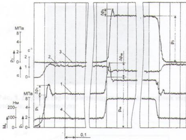
Рис. 5. Осцилограма перехідних процесів вмонтованого гідравлічного приводу конвеєра, чутливого до навантаження, за тиску відкриття p_{zv}=12 МПа, крутильної жорсткості c_p=0,37 \cdot 10^{-3} Н·м/рад; f_3/f_4=0,6 : 1 — зміна тиску в напірній гідромагістралі першого гідромотора; 2 — зміна частоти обертання виконавчої ланки приводу; 3 — зміна тиску в напірній гідромагістралі другого гідромотора; 4 — зміна навантаження (східчаста) на виконавчій ланці приводу
