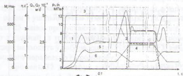
Рис. 4. Теоретичні залежності p_1(t), p_3(t), Q_1(t), Q_2(t), n(t), M(t) (криві 1 — 6 відповідно) від часу: p_{кз}=12 МПа; c_p=0,37 \cdot 10^{-3} Н·м/рад; f_3/f_4=0,6 ; трапецеїдальна зміна навантаження
