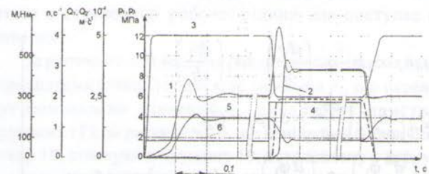
Рис. 3. Теоретичні залежності p_1(t), p_3(t), Q_1(t), Q_2(t), n(t), M(t) (криві 1 — 6 відповідно) від часу: p_{кз}=12 МПа; c_p=0,37 \cdot 10^{-3} Н·м/рад; f_3/f_4=0,6 ; східчаста зміна навантаження
