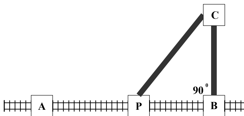
Рис.1 Геометричне тлумачення задачі
