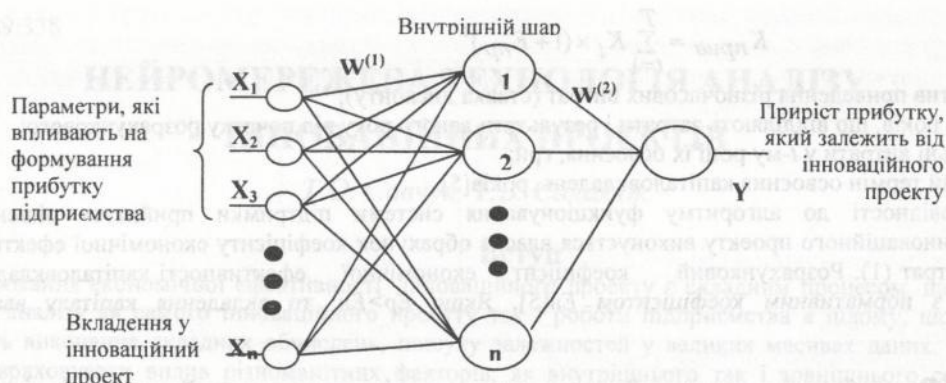
Рисунок 2 - Структура нейронної мережі
