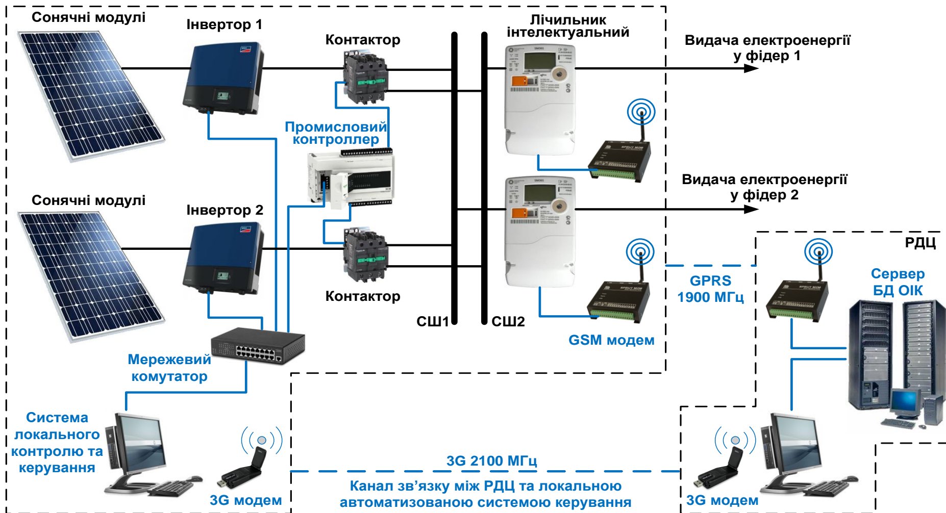
Рис. 2 – Особливості апаратної реалізації АСК схемою видачі потужності ВДЕ
