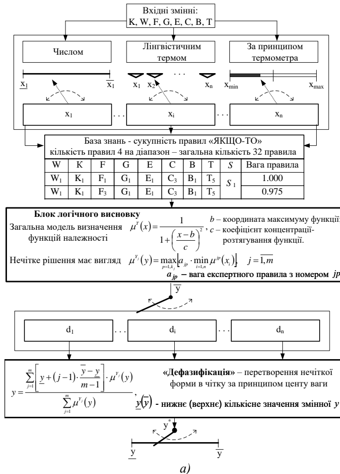
Рисунок 3 – Блок схема апроксимації визначення дальності видимості (а) та її реалізація у вигляді комплексної програми (б, в): б – форма для введення вихідних даних; в – форма перетворення нечіткої інформації в чітку за принципом «центру ваги» – дефазифікація
