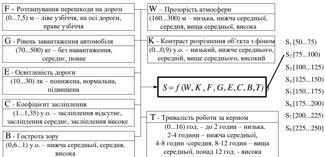
Рисунок 2 – Структура програми для визначення дальності видимості (фактори впливу, універсальна множина та терми для їх оцінок)
