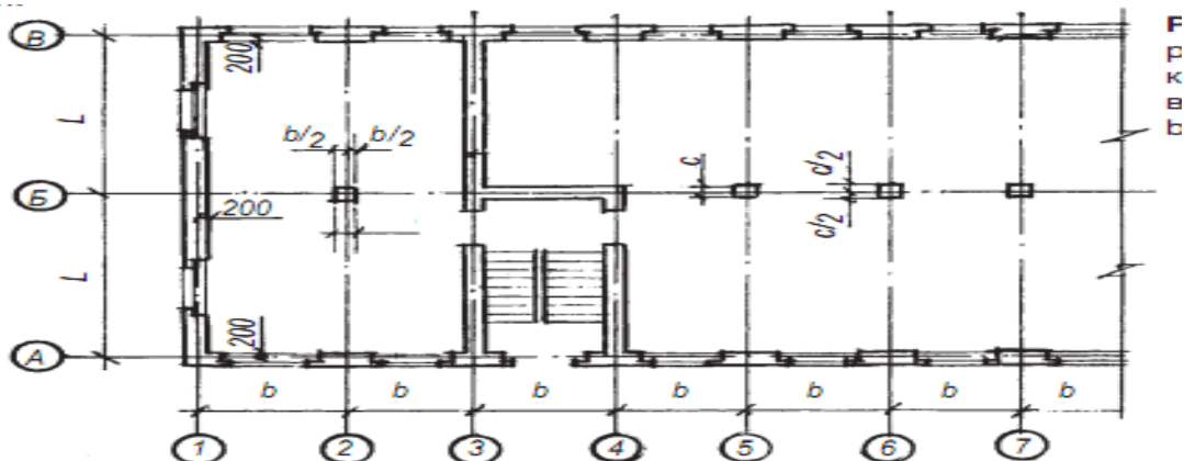
Рисунок 4 – Схема розташування маркувальних осей у плані будинку:
