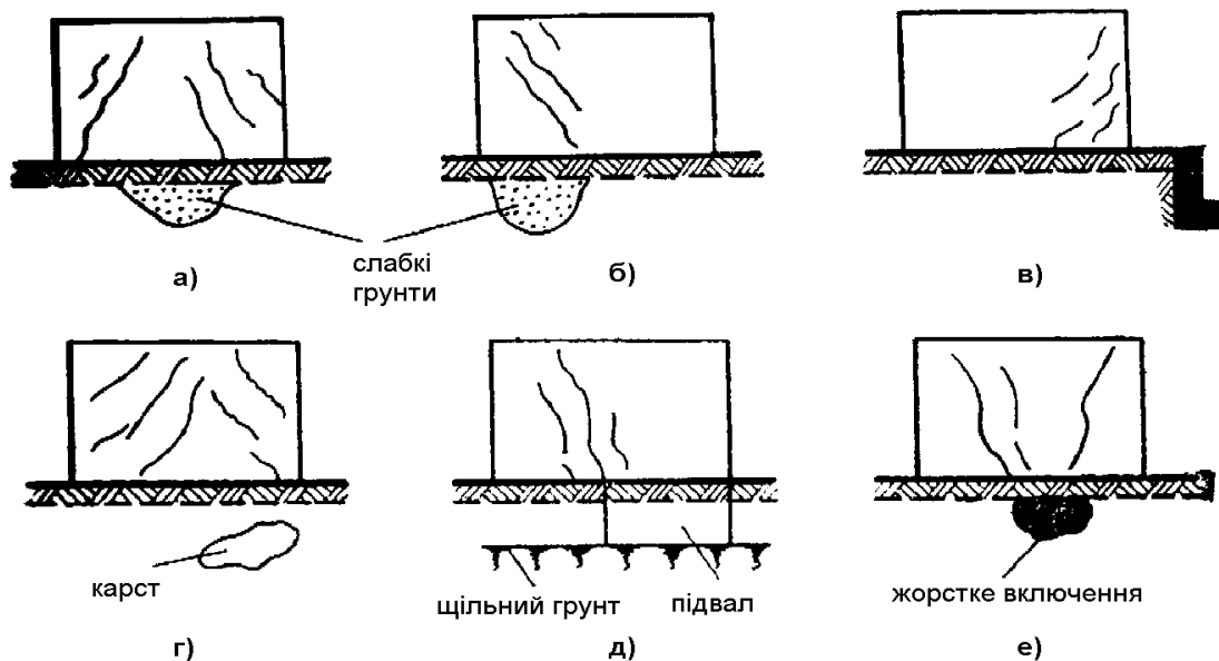
Рис. 1.1. Осадові тріщини [74]
