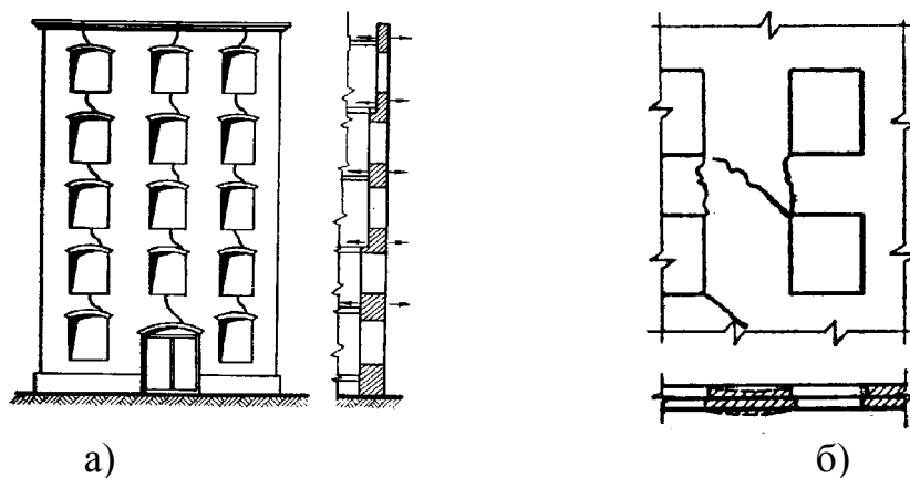
Рис. 1.2. Силлові тріщини [74]
