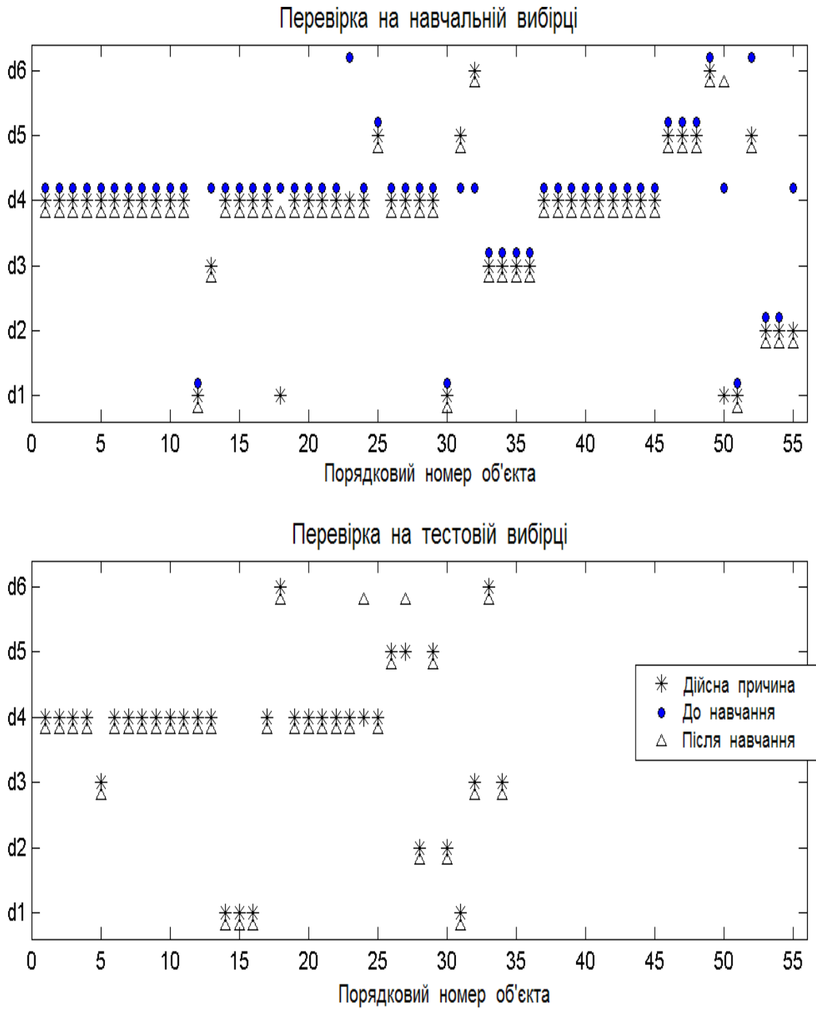
Рис. 3.2. Перевірка діагностичної моделі
