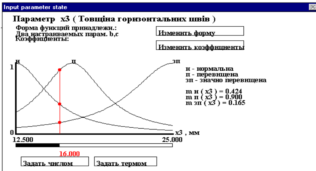
Рис. 3.6. Вікно функцій належності
