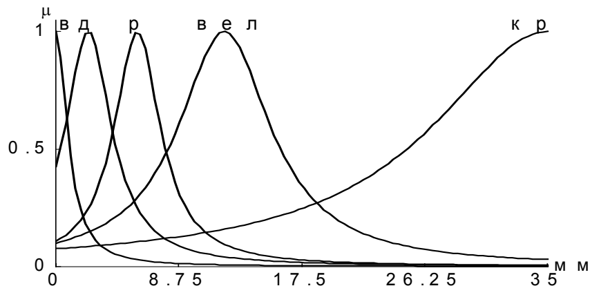
Рис. 2.2. Приклад функцій належності
