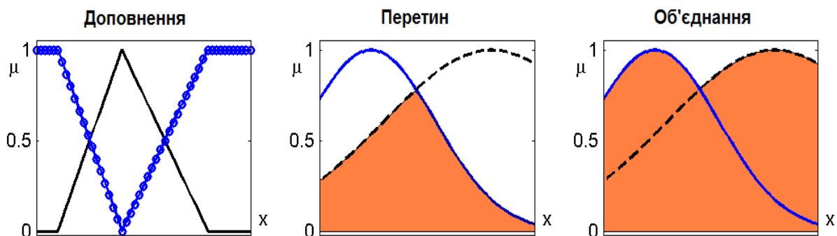
Рис. 2.1. Операції над нечіткими множинами
