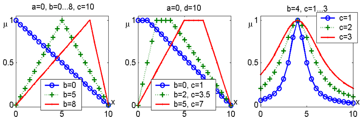
Рис. 2.5. Популярні функції належності
