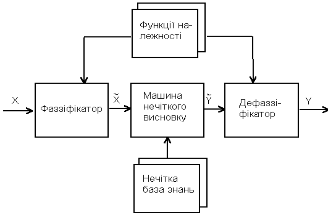
Рис. 2.6. Типова архітектура системи нечіткого висновку
