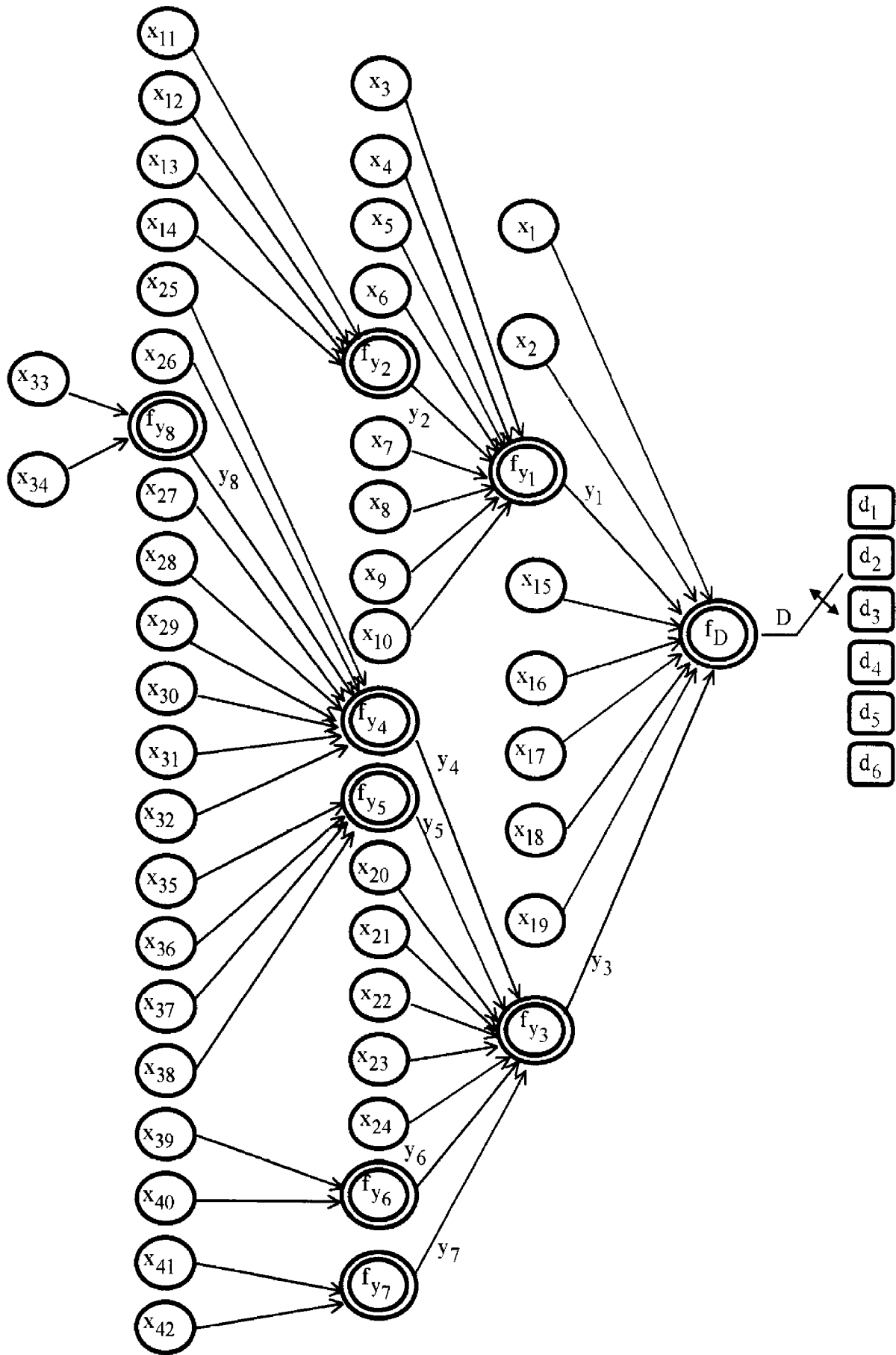
Рис. 3.1. Дерево логічного висновку для діагностування тріщини
