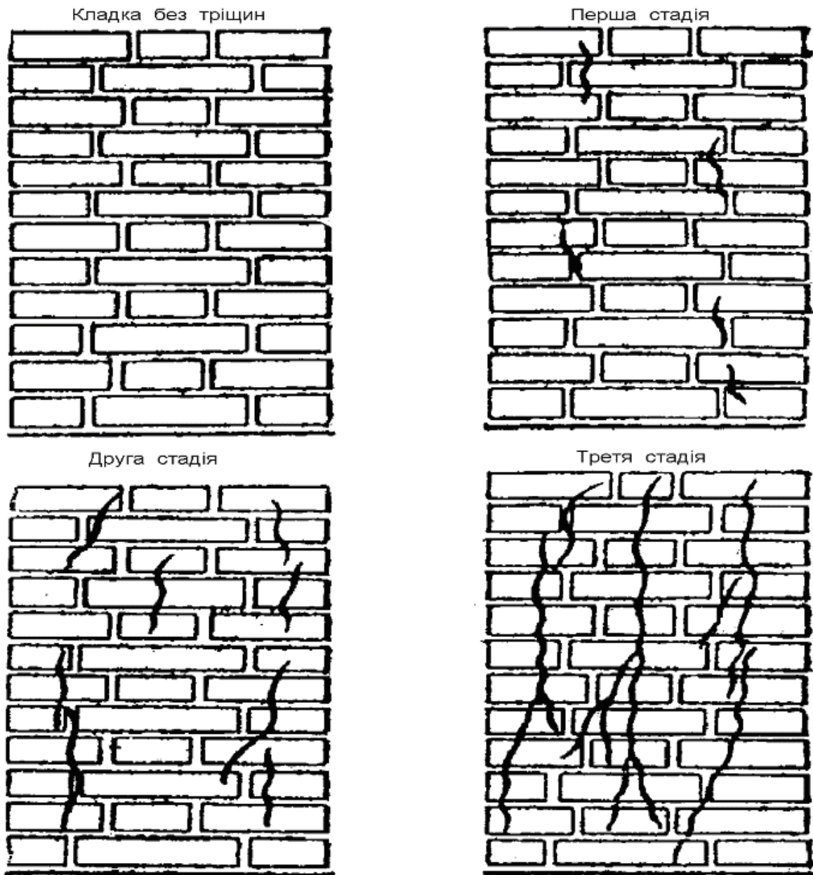
Рис. 1.4. Стадії тріщиноутворення в цегляній кладці [3]
