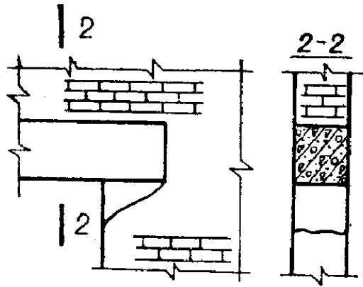
Рис. 1.3. Тріщина від усадки монолітної перемички [74]
