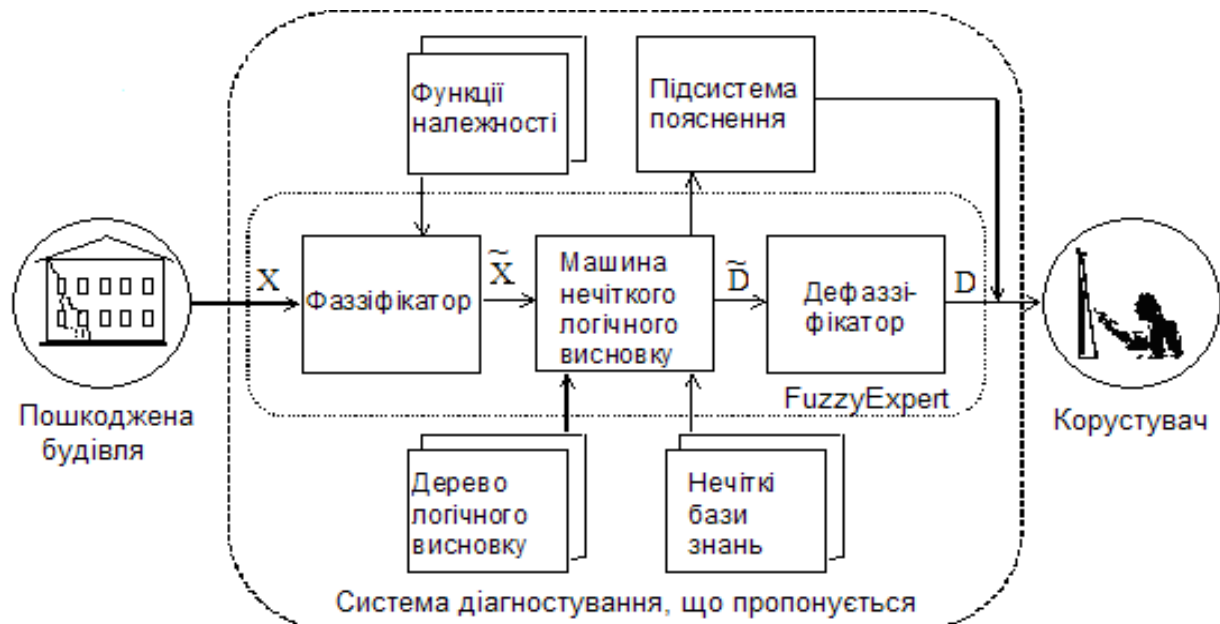
Рис. 3.4. Архітектура автоматизованої системи діагностування
