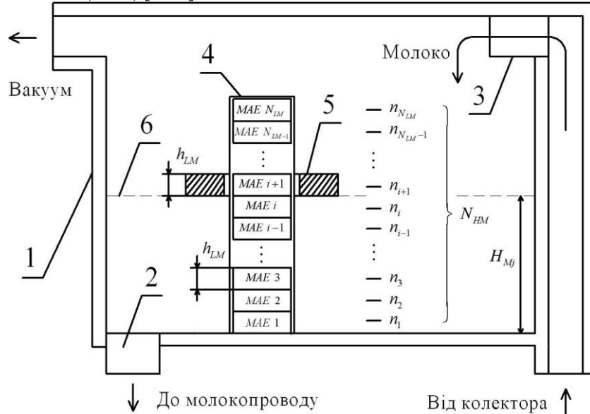
Рис. 2. Схематичне креслення молокоприймальної камери доїльного апарата з вимірювальним перетворювачем рівня молока з дискретним вихідним сигналом на основі МАЕ:
