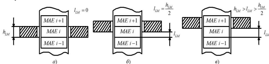
Рис. 3. Варіанти взаємного розташування МАЕ та поплавка з магнітом
