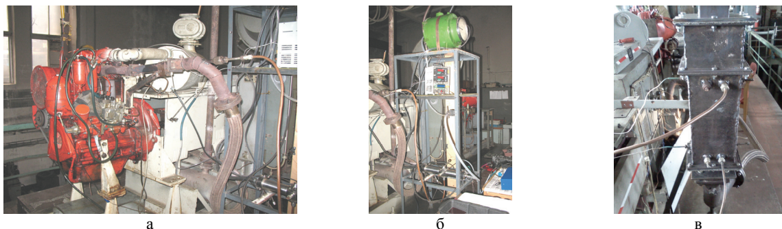
Рис. 2. Модернізована випускна система МВС, обладнана МВ і системою відбору проб ВГ на токсичність і димність: а — загальний вигляд; б — стоек з приладами; в — макетоутримувальна вставка
