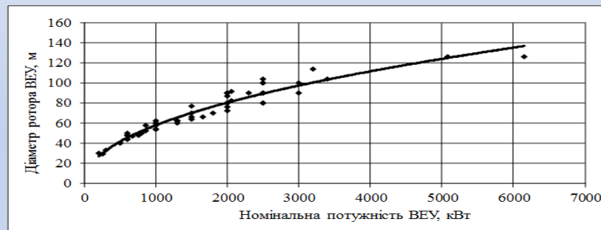
Рисунок 9.2 – Залежність діаметра ротора від потужності ВЕУ
