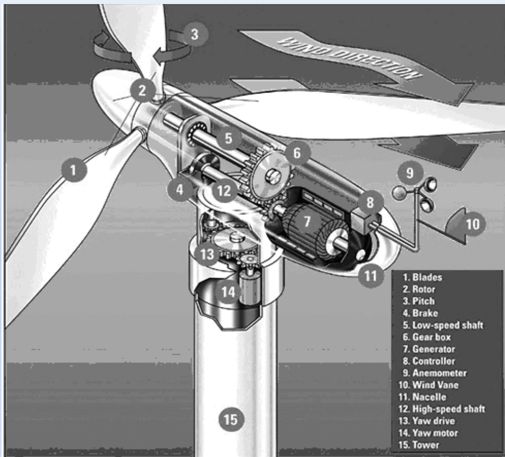
Рисунок – 5.1. Конструкція вітрової електричної установки:
