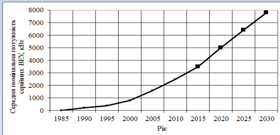
Рисунок 9.1 – Спостережені і прогнозні значення середньої світової номінальної потужності введених в експлуатацію наземних ВЕУ
