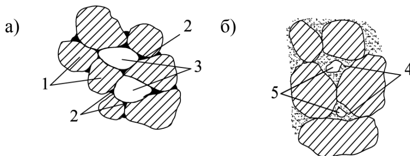
Рис. 3. Схеми стану капілярної вологоємності: а) капілярно-стиковий; б) капілярно-четочний: 1 – мінеральні частинки; 2 – капілярно-стиковий стан (затиснена вода); 3 – вільний газ; 4 – капілярно-четочний стан; 5 – затиснений газ в порах
