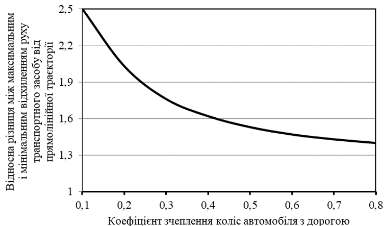
Рисунок 2 – Зміна похибки розрахунку відхилення транспортного засобу в напрямку перпендикулярному початковому напрямку руху від коефіцієнта зчеплення колеса з дорогою
