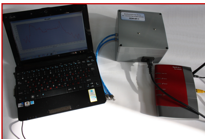
Рисунок 1 – Фото приладу RDM-BP-1
