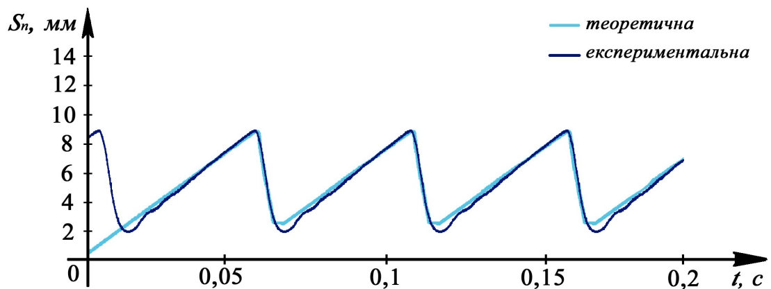
Рис. 3. Зведений графік теоретичного та експериментального переміщення поршня гідроциліндра S_n
