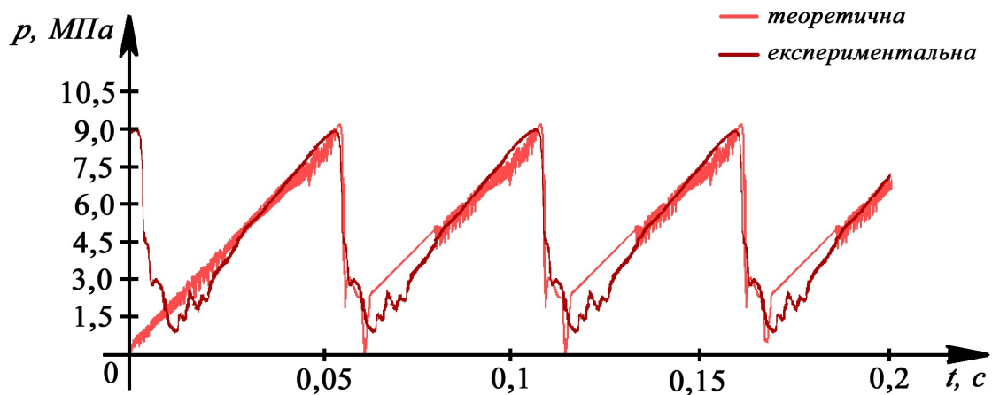
Рис. 2. Зведений графік зміни тиску в гідроциліндрі P(t)
