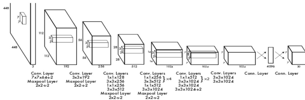
Рис. 1. Послідовність та розміри прихованих шарів розробленої мережі
