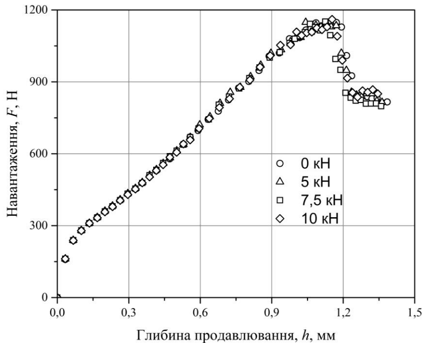
Рис. 4. Діаграми деформування дискового мікрозразка із сталі 45 за різних зусиль затиску зразка
