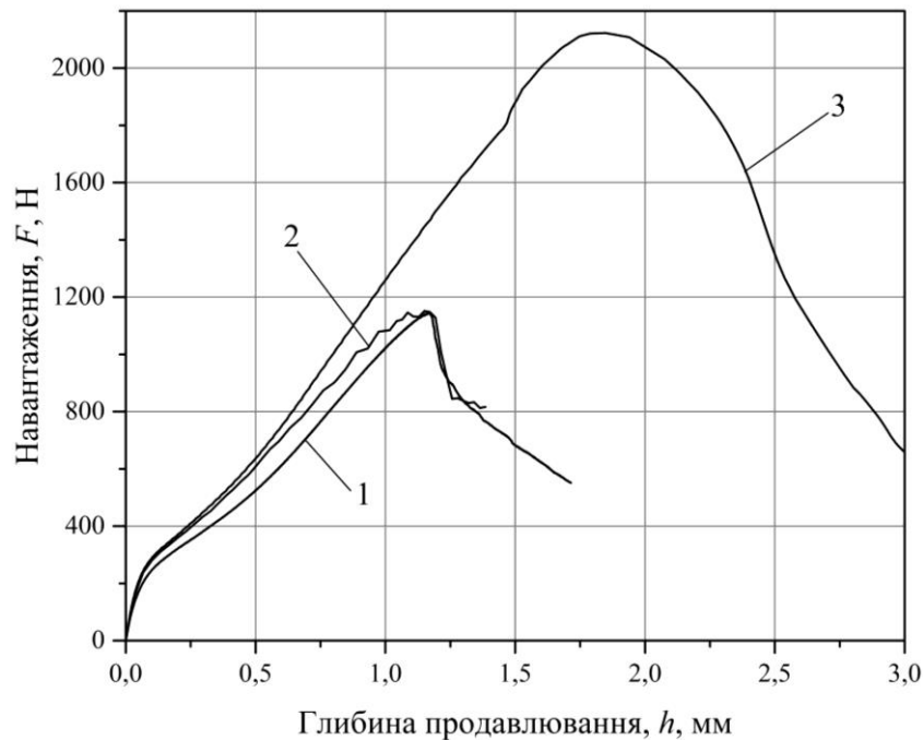
Рис. 3 Експериментальна (1) та розрахункові діаграми деформування дискових мікрорізків з урахуванням моделі GTN (2) та без (3).
