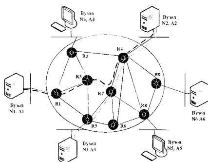
Рисунок 2.9 – Принцип роботи віртуального каналу
