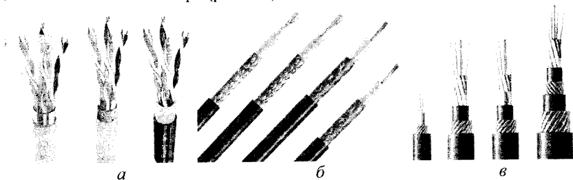
Рисунок 4.3 – Кабелі зв'язку: a – кабелі на основі крученої пари; б – коаксіальні; в – волоконно-оптичні
