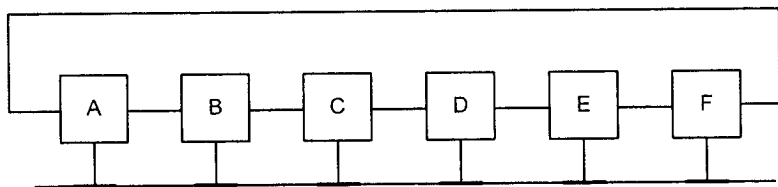
Рисунок 2.13 – Фізична топологія загальна «шина» та логічна «кільце»
