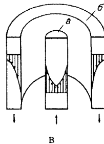
Рисунок 4.18 – Електричні процеси у коаксіальній парі: a – взаємодія магнітних полів провідників пари; б – лінії електромагнітних полів між провідниками пари; в – щільність розподілу струмів на взаємно обернених поверхнях провідників пари
