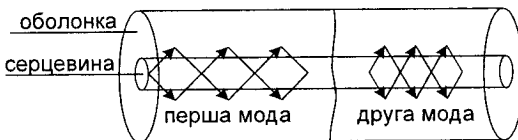
Рисунок 4.10 – Поширення різних мод у оптичному волокні
