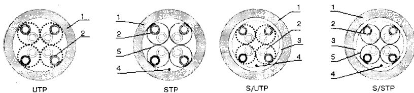
Рисунок 4.17 – Екранована і неекранована кручена пара:
