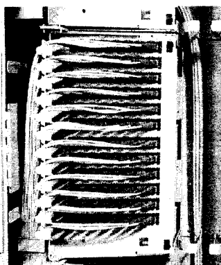
Рисунок 4.5 – Кінцеві пристрої ліній зв'язку: а – оптичні панелі ODF у телекомунікаційній шафі; б – електричні плінти DDF у навісному настінному боксі
