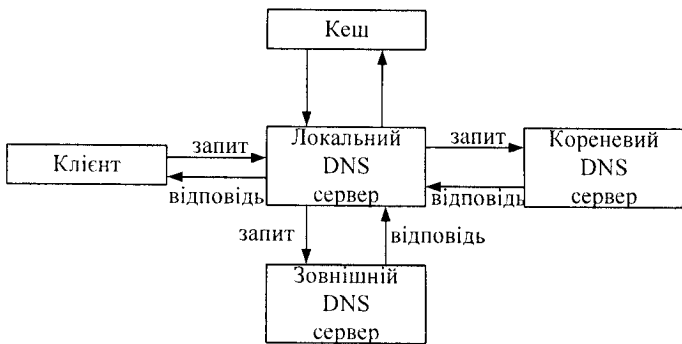
Рисунок 5.4 – Запити в системі DNS
