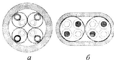
Рисунок 4.16 – Види скручування кручених пар: а – парна; б – четвіркова
