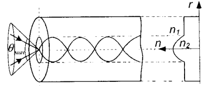
Рисунок 4.9 – Оптичне волокно із градієнтним профілем показника заломлення
