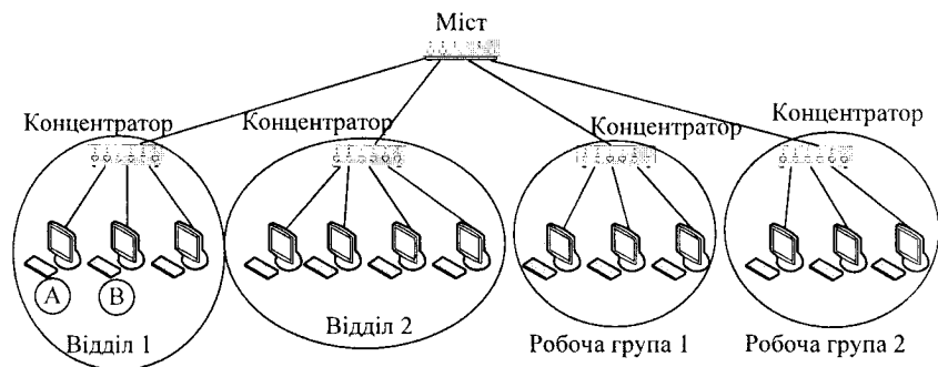
Рисунок 2.16 – Мережа після логічної структуризації
