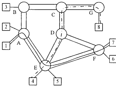
Рисунок 2.7 – Загальна структура мережі з комутацією абонентів
