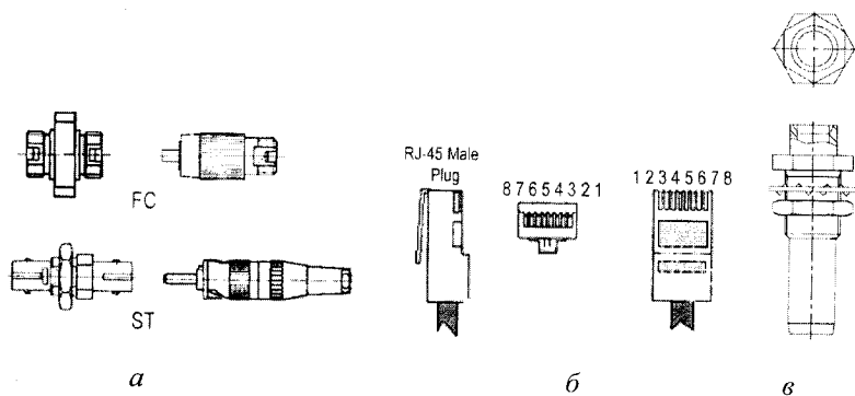
Рисунок 4.6 – Роз'ємні з'єднання ліній зв'язку: а – оптичні роз'єми FC та ST; б – роз'єм RJ-45 крученої пари; в – коаксіальний роз'єм BMA
