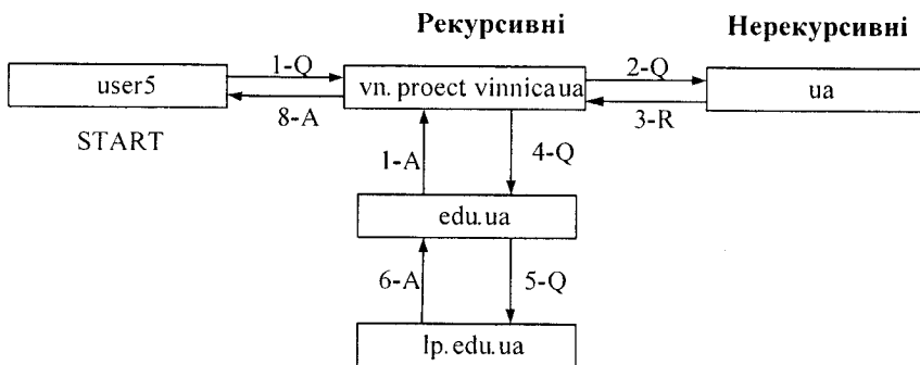
Рисунок 5.5 – Процес обробки запиту в DNS, де Q – запит, А – відповідь, R – посилання
