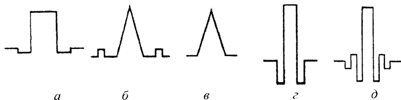
Рисунок 4.13 – Профілі показників заломлення оптичних волокон
