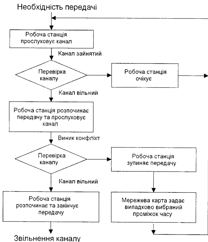
Рисунок 2.6 – Алгоритм методу CSMA/CD
