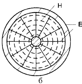
Рисунок 4.18 – Електричні процеси у коаксіальній парі: a – взаємодія магнітних полів провідників пари; б – лінії електромагнітних полів між провідниками пари; в – щільність розподілу струмів на взаємно обернених поверхнях провідників пари
