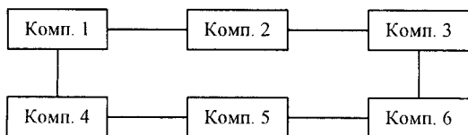
Рисунок 2.4 – Топологія «кільце»
