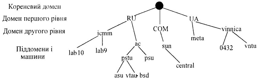
Рисунок 5.3 – Доменна структура імен
