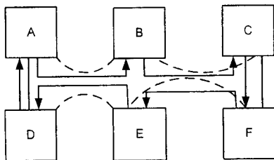
Рисунок 2.12 – Фізична топологія «кільце» та логічна «кільце»
