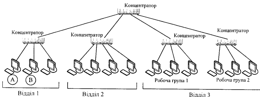
Рисунок 2.15 – Мережа після фізичної структуризації
