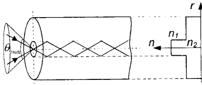
Рисунок 4.8 – Оптичне волокно із ступінчастим профілем показника заломлення
