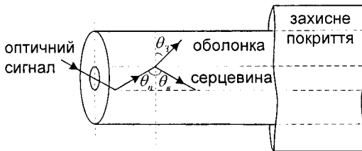
Рисунок 4.7 – Структура оптичного волокна
