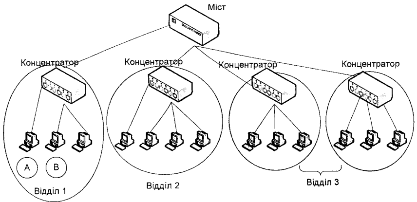
Рисунок 4.22 – Єдине роздільне середовище за допомогою моста перетворене на чотири роздільних середовища
