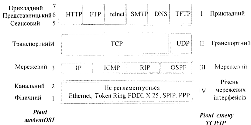
Рисунок 5.1 – Стек протоколів TCP/IP
