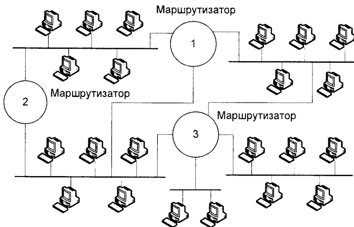
Рисунок 4.24 – Комірчаста мережа з маршрутизаторами
