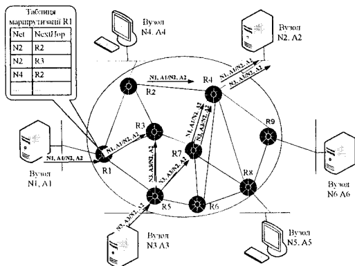
Рисунок 2.10 – Дейтаграмний принцип передачі пакетів
