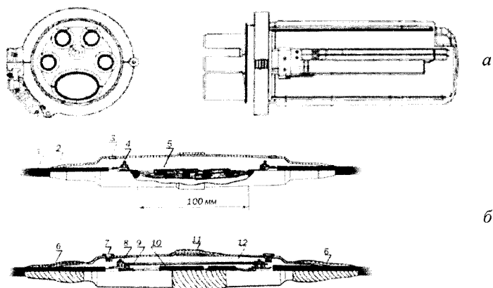
Рисунок 4.4 – Муфти кабельних ліній зв'язку: а – муфта FOSC-400A4 для оптичних кабелів; б – муфта МП для симетричних кабелів
