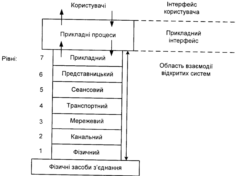
Рисунок 3.1 – Модель OSI
