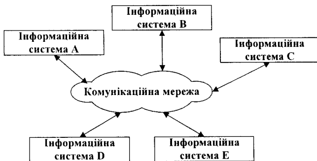
Рисунок 1.1 – Однорангова архітектура
