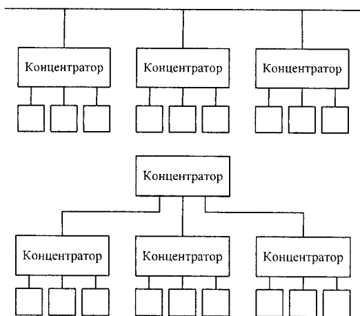
Рисунок 2.5 – Комбіновані топології
