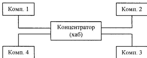
Рисунок 2.3 – Топологія «зірка»
