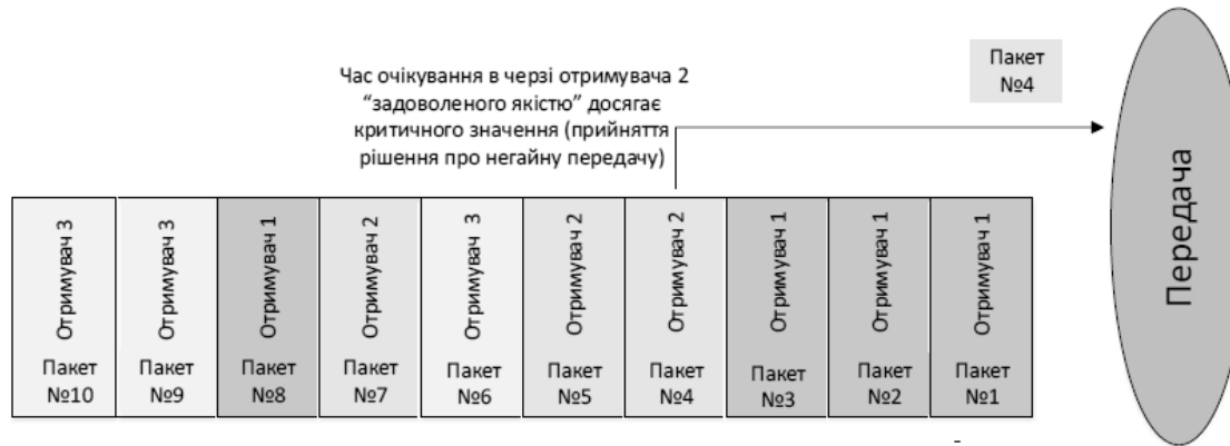
Рисунок 2 – Принцип роботи модифікованого алгоритму вибору пакета
