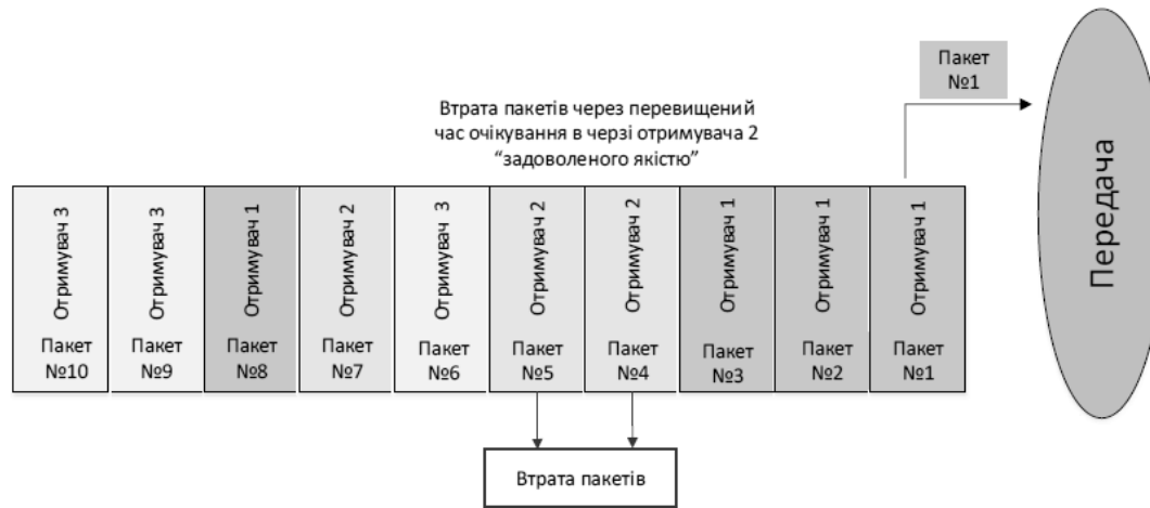
Рисунок 1 – Принцип роботи існуючого алгоритму вибору пакета
