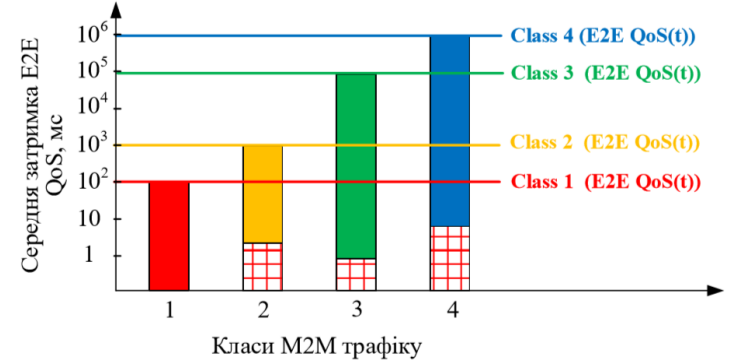
Рисунок 2 – Середня затримка обслуговування після оптимізації
