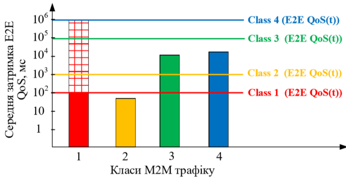
Рисунок 1 – Середня затримка обслуговування до оптимізації
