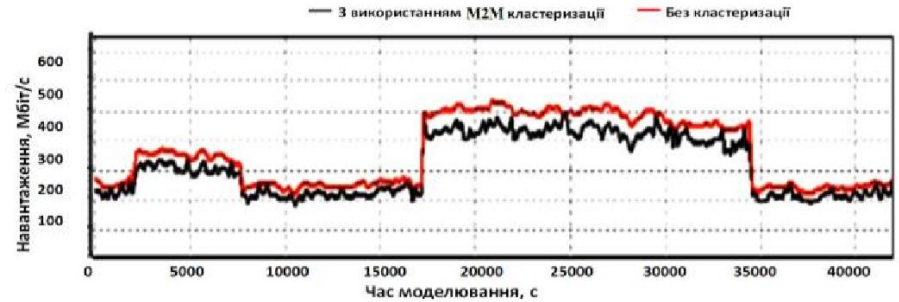
Рисунок 3 – Навантаження на мережу з кластеризацією і без кластеризації
