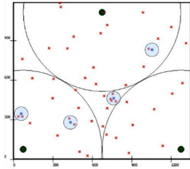
Рисунок 1 – Структура мережі при малому навантаженні
