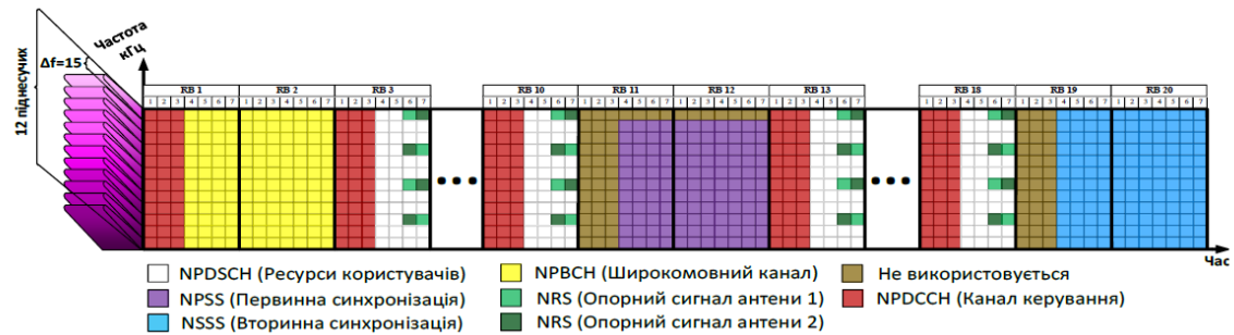
Рисунок 1 – Розташування корисних та сигналізаційних та даних у низхідному каналі
