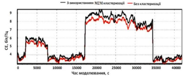
Рисунок 4 – Системна спектральна ефективність
