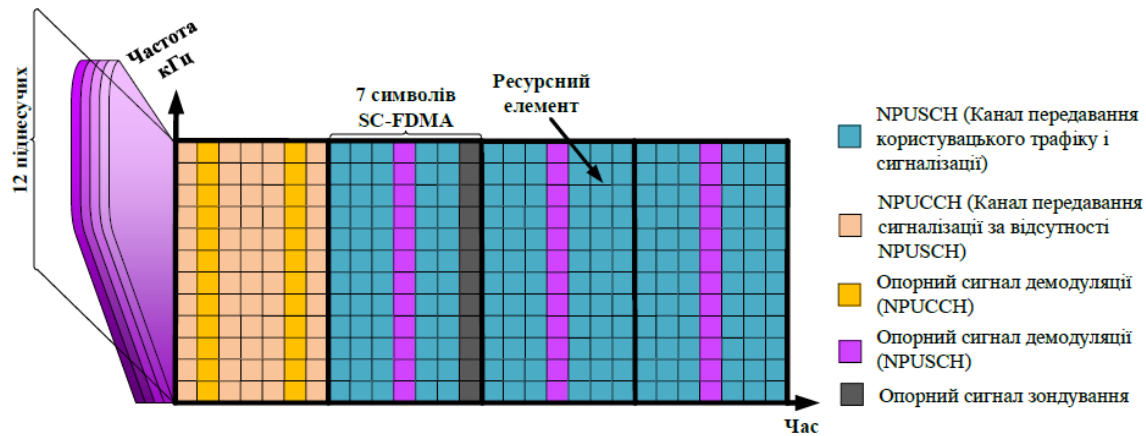
Рисунок 2 – Розташування корисних та сигналізаційних та даних у висхідному каналі
