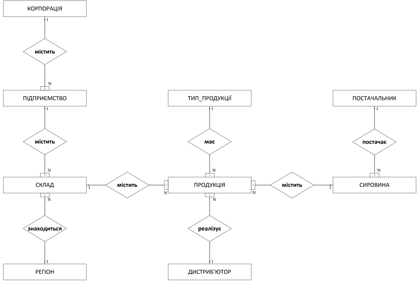
Рисунок 3 – ER-модель для бази даних пивоварної продукції України
