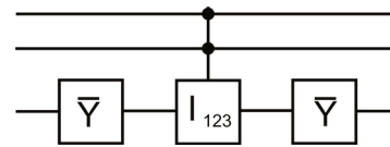
Fig. 5. XOR gate
