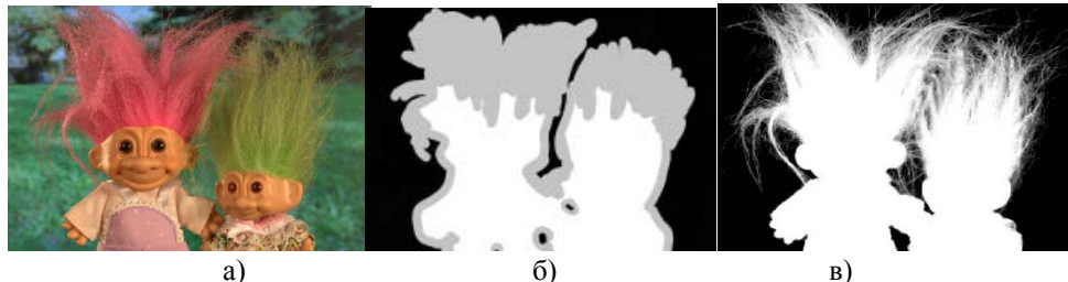
Рис. 1. Вхідні та вихідні данні (а – вхідне зображення, б – вхідний тримап, в – карта прозорості зображення).
