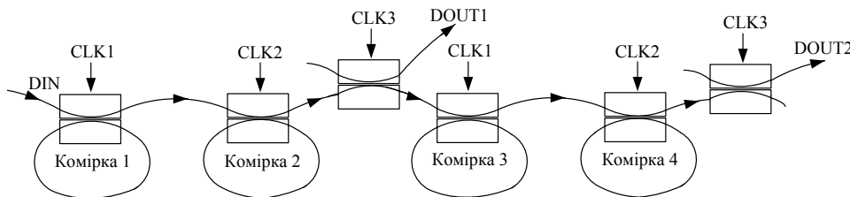
Рис. 5. Двохрозрядний перетворювач послідовного коду в паралельний
