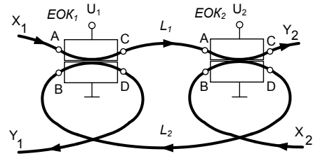
Рис. 2. Схема волоконно-оптичного запам'ятовуючого пристрою з використанням електрооптичних \text{LiNbO}_3 комутаторів
