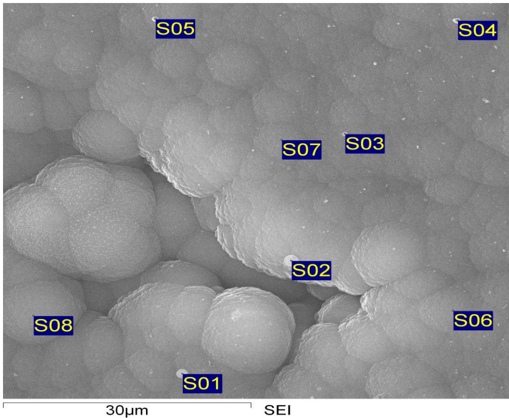
Рисунок 7.2 – Фотографія поверхні нанесеного покриття методом електронно-променевого випаровування та осадження (електронно-променевий мікроскоп)
