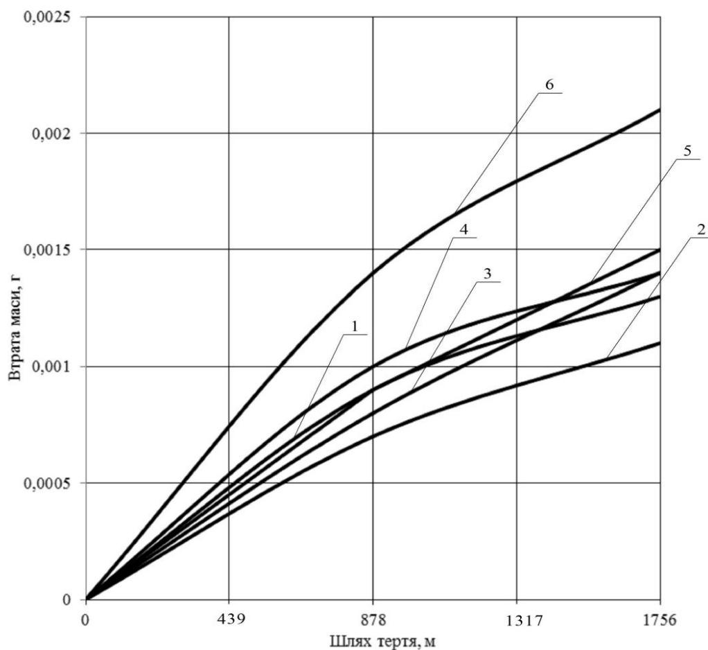
Рисунок 4.10 - Кінетика зношування високовуглецевих покриттів наплавлених на швидкостях: 1) V_{\text{напл}}=11 м/год; 2) V_{\text{напл}}=14 м/год; 3) V_{\text{напл}}=17 м/год; 4) V_{\text{напл}}=20 м/год; 5) V_{\text{напл}}=23 м/год; 6) V_{\text{напл}}=26 м/год.
