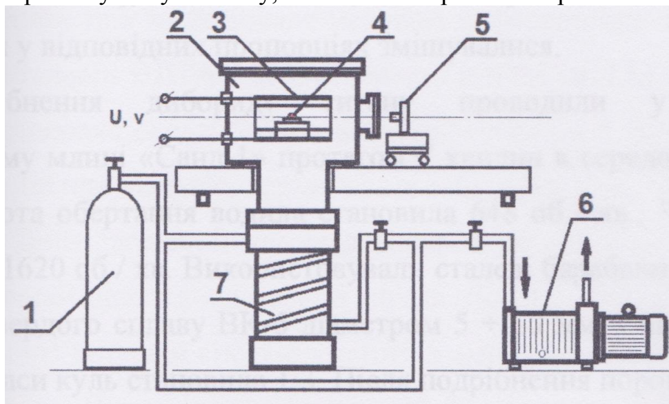
Рисунок 3.2 – Установка для визначення кінетики розтікання:
