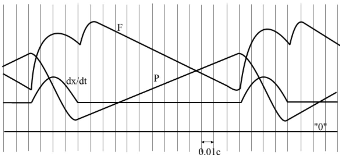
Рисунок 4.2 – Приклад типової осцилограми руху з релаксаційними коливаннями
