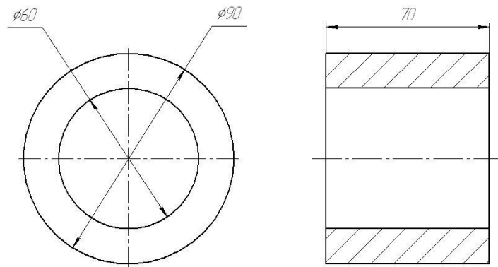
Рисунок 2.3 – Зразки для досліджень операції наплавлення
