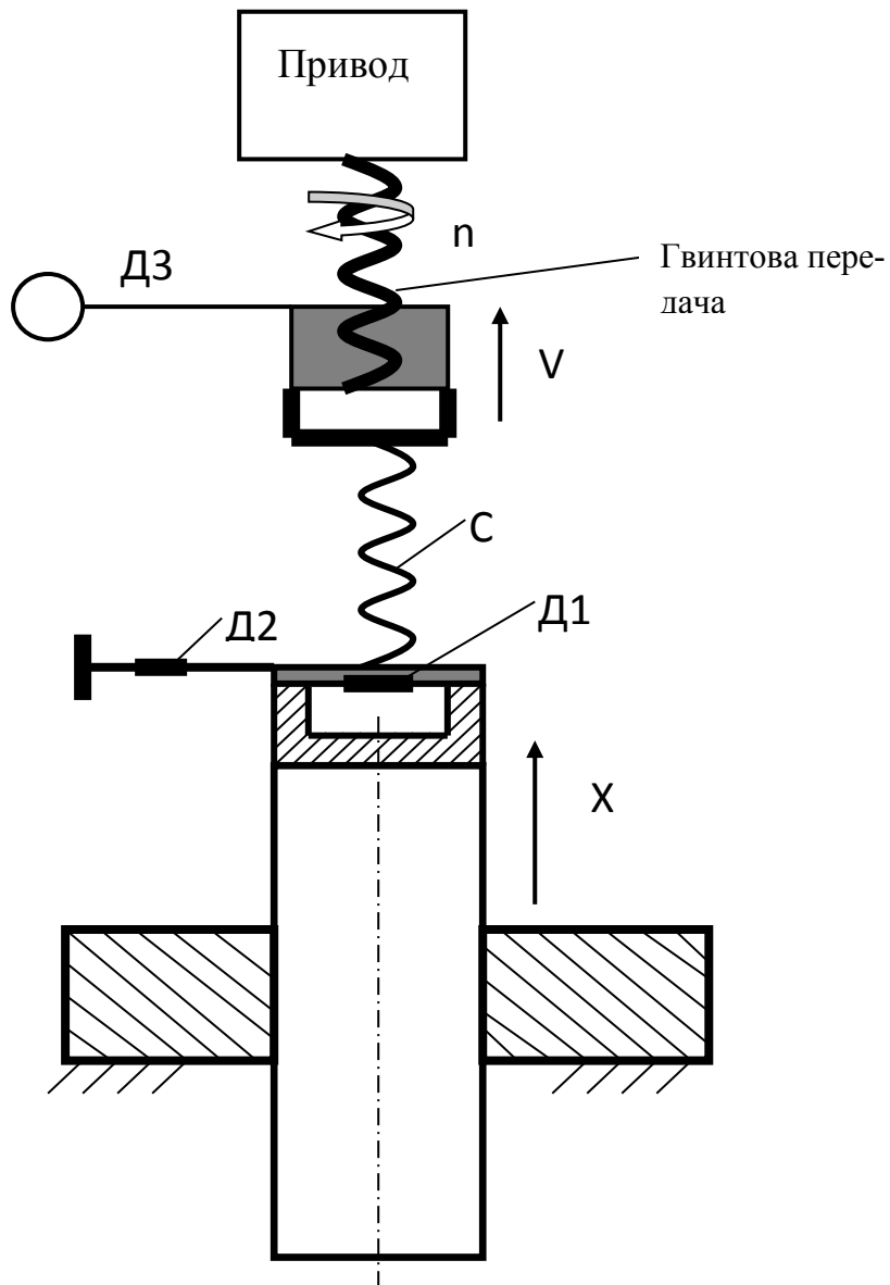
Рисунок 4.1 – Установка для експериментального визначення коефіцієнтів тертя спокою
