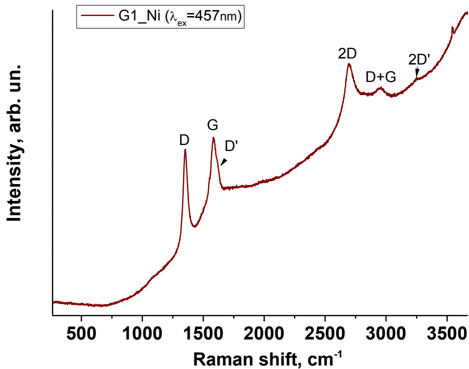
Рисунок 2.9 – Приклад раманівського спектру тонких вуглецевих плівок
