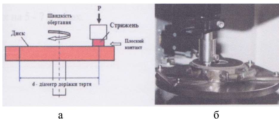
Рисунок 4.8 - Схема випробувань (а) і вигляд вузла тертя (б) на трибо-тестері Bruker UMT Multi-Specimen Test System
