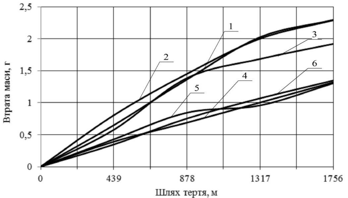
Рисунок 4.11 – Кінетика зношування контртіла з сталі 45 при таких швидкостях наплавлення: 1) V_{\text{напл}}=11\text{м/год} ; 2) V_{\text{напл}}=14\text{м/год} ; 3) V_{\text{напл}}=17\text{м/год} ; 4) V_{\text{напл}}=20\text{м/год} ; 5) V_{\text{напл}}=23\text{м/год} ; 6) V_{\text{напл}}=26\text{м/год}
