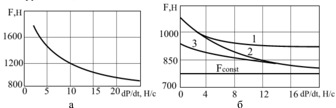
Рисунок 4.4 – Вплив на силу тертя спокою швидкості наростання зсувної сили (ковзання без мастила)
