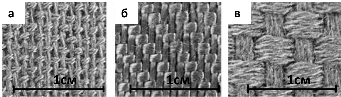
Рисунок 2.1 – Вуглецеві тканини марки УУТ-2: щільність 150 г/м 2 (а), 200 г/м 2 (б), 250г/м 2 (в)
