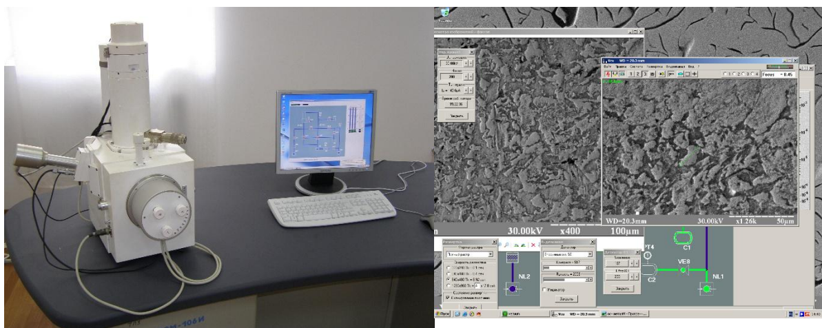
Рисунок 2.8 – Електронний мікроскоп РЕМ-106И
