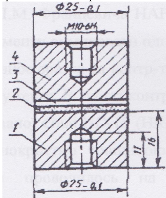
Рис. 3.3 Зразок з покриттям, склеєний з контртілом для випробувань на адгезійну міцність: 1 - зразок з покриттям; 2 - покриття; 3 - прошарок клею; 4 - контртіло.
