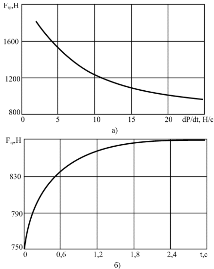
Рисунок 4.5 – Статичні характеристики тертя (трибоконтакт з мастилом):
