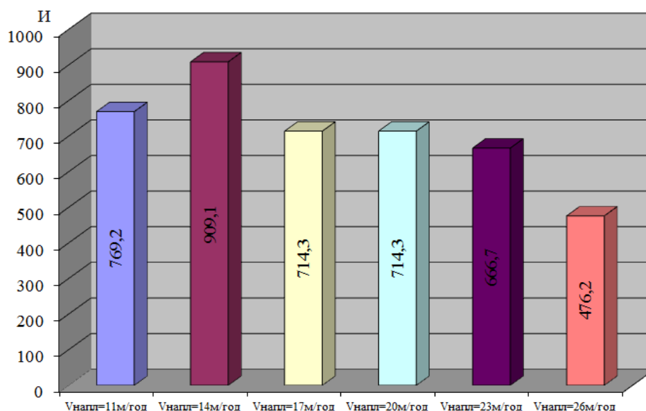
Рисунок 4.12 - Зносостійкість високовуглецевого покриття при зміні швидкості наплавлення
