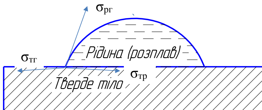
Рисунок 3.1 – Схема векторів поверхневих натягів \sigma_{\text{ТГ}} , \sigma_{\text{РГ}} і \sigma_{\text{ТР}} для системи «тверде тіло - рідина»
