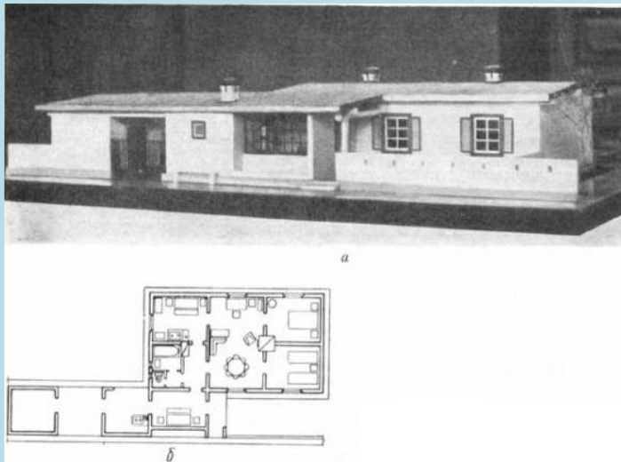
Проект індустріально-збірного житлового будинку для Донбасу, 1948р.
