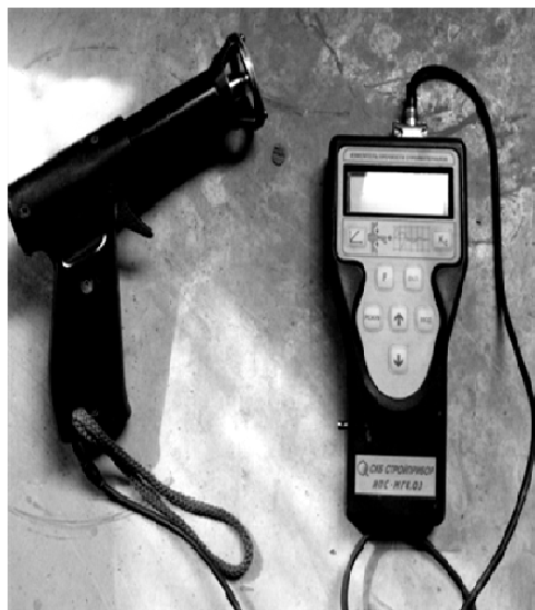
Рисунок 5 – Вимірювач міцності будматеріалів ИПС МГ4.03 (СКБ Стройприбор, м. Челябинськ)
