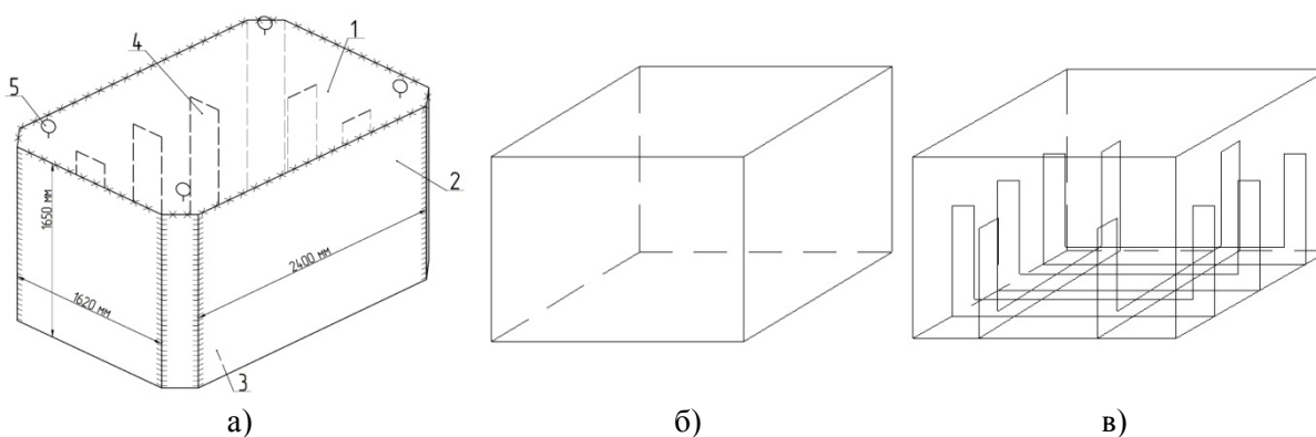
Рис. 1. Контейнер: а – загальний вигляд, де 1 – кришка, 2 – стінка, 3 – дно, 4 – ребра жорсткості, 5 – рим-болт; б – схема контейнера без ребер жорсткості (стандартне рішення); в – схема контейнера з ребрами жорсткості (пропонується)
