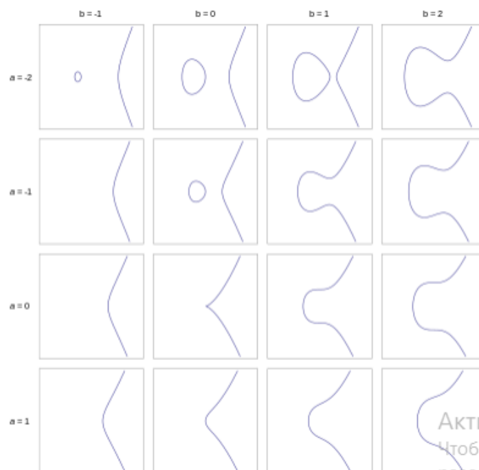
Рисунок 1 – приклад еліптичних кривих
