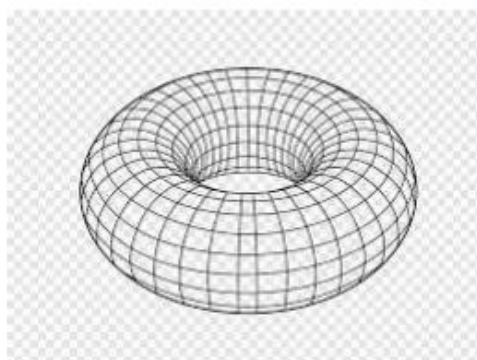
Рисунок 2 – приклад топології та геометрії
