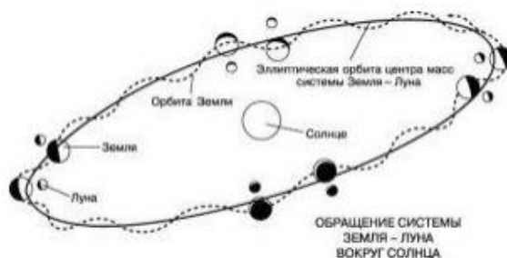
Рисунок 5 – приклад планети, яка рухається під дією гравітаційного поля
