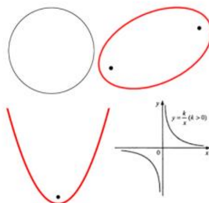
Рисунок 3 – приклад кола, еліпси, параболи та гіперболи
