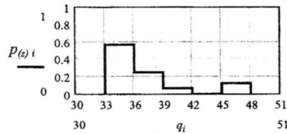
Рис.1 – Гістограма вариційного ряду вибірки електроспоживання трамваями за годину
