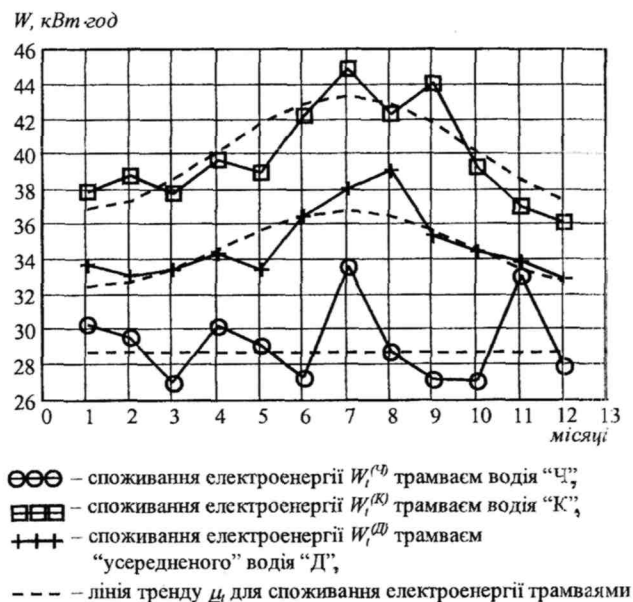
Рис.3 – Споживання електроенергії трамваєм протягом досліджуваного періоду
