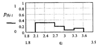
Рис.2 – Гістограма вариційного ряду вибірки електроспоживання трамваями на 1 км
