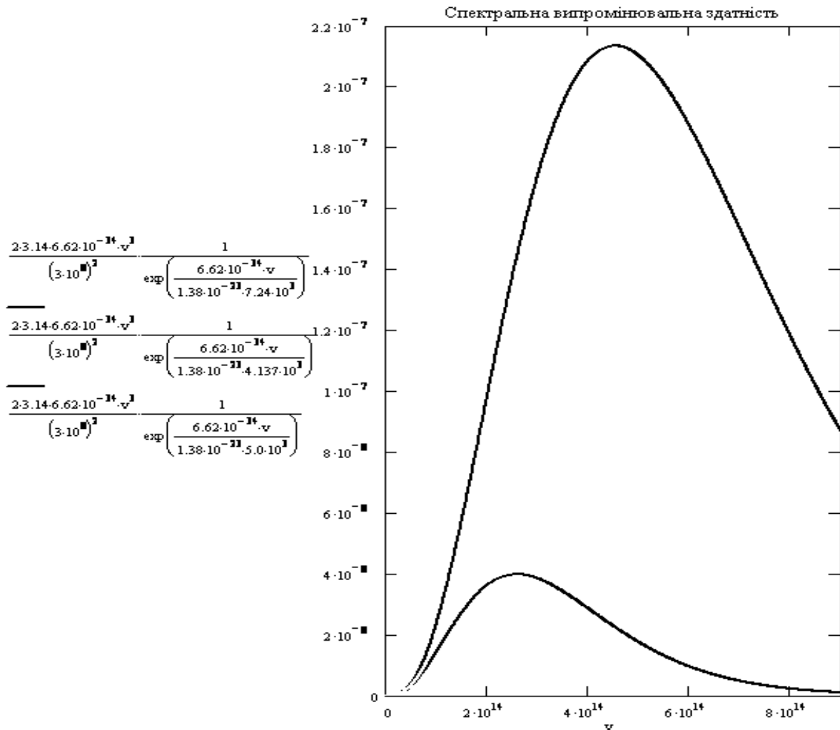
Рис. 1. Розподіл енергії випромінювання за частотою \nu та температурою T
