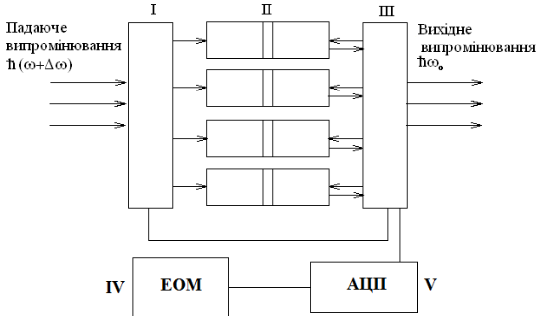
Рис. 2. Блок-схема спектротрансформатора
