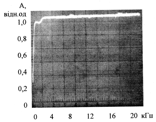
Рис. 4. Амплітудно-частотна характеристика: а) 1 — для R = 10 кОм, 2 — для R = 1 кОм (комп'ютерне моделювання в пакеті MathCAD 2001); б) експериментально отримана АЧХ
