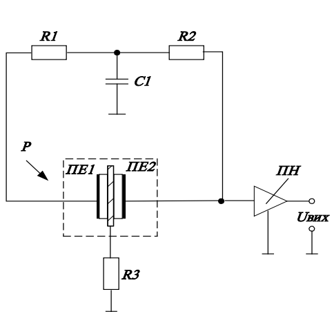
Рис. 5. Перетворювач механічних величин з триморфним п'єзоелементом в схемі режекторного фільтра: а) подвійна Т-подібна мостова схема з'єднання; б) експериментально отримана АЧХ
