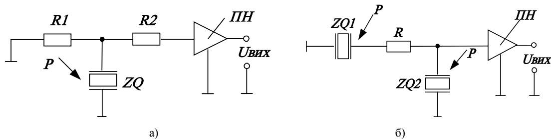
Рис. 1. Перетворювач механічних величин з п'єзоелементами в схемі фільтра нижніх частот: а) Т-подібна схема з'єднання; б) Г-подібна схема з'єднання
