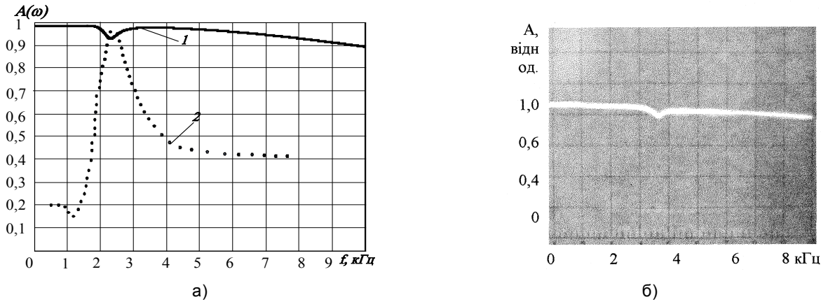
Рис. 2. Амплітудно-частотна характеристика: а) 1 — крива запропонованого перетворювача, 2 — крива п'єзоелектричного перетворювача (комп'ютерне моделювання в пакеті MathCAD 2001); б) експериментально отримана АЧХ
