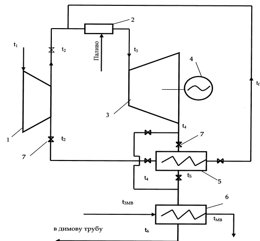
Принципова теплова схема ГТУ-ТЕЦ:
