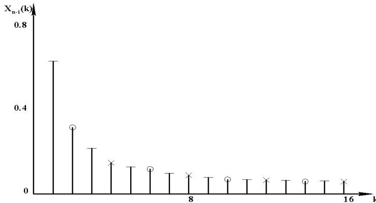
Рис. 2. Частотні спектри підпоследовностей, що відображають інтегральні нелінійності 4-розрядного АЦП
