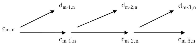
Вейвлет перетворення
