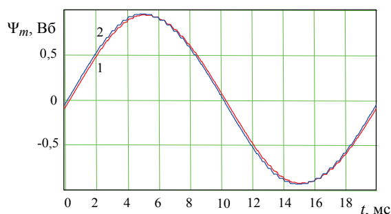
Рис. 7. Залежності потокозчеплення, що розраховані за формулами (5) та (6) за наявності похибки визначення R'_r
