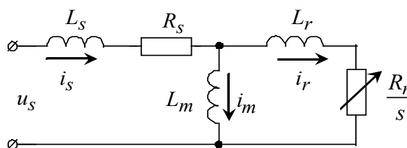
Рис. 1. Т-подібна схема заміщення асинхронного двигуна
