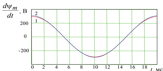
Рис. 2. Залежності похідної потокозчеплення, що розраховані за формулами (3) і (4)
