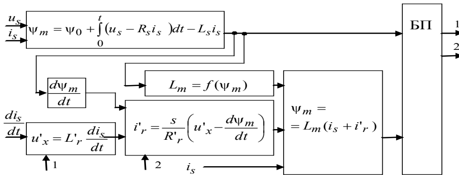
Рис. 3. Функціональна схема перетворень за формулами (5) і (6)
