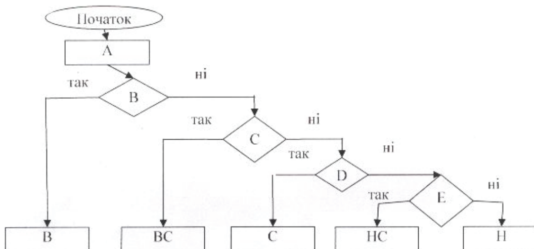
Рис. 1. Граф-схема оцінювання якісних параметрів x_{11}, x_{12}, x_{13}, x_{14}, x_{22}, x_{23}, x_{34}, x_{35}, x_{41}, x_{42}, x_{71} t -м лінгвістичним термом, t = \overline{1, T} , T = 5
