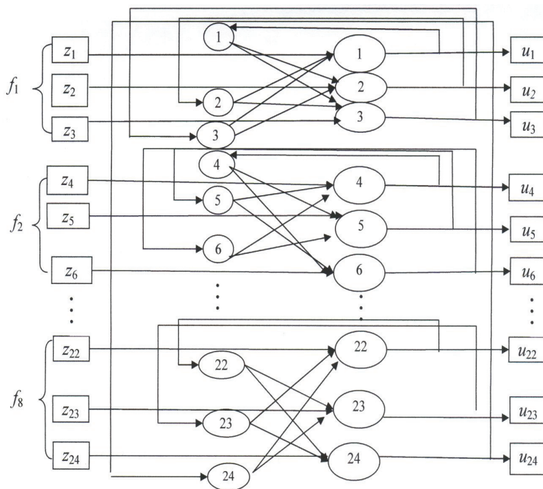
Рис. 2. Структура нейронної мережі Хопфілда для оцінювання СПП
