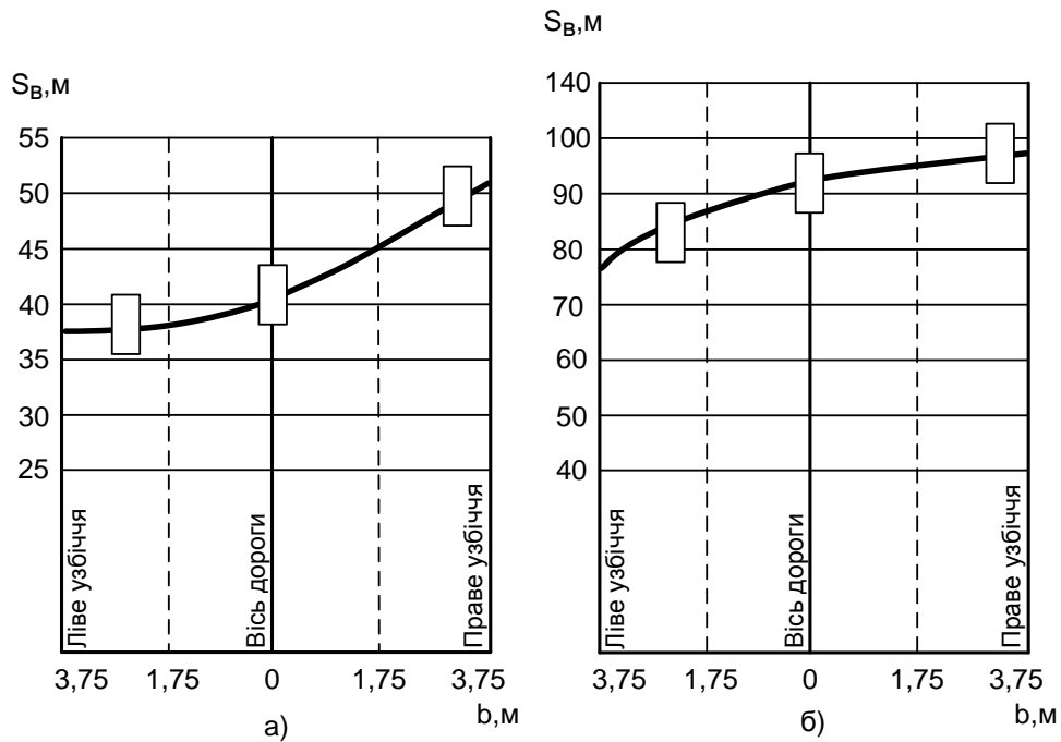
a – ближнє світло фар; б – дальнє світло фар Рис. 5. Залежність дальності видимості від розташування перешкоди на дорозі
