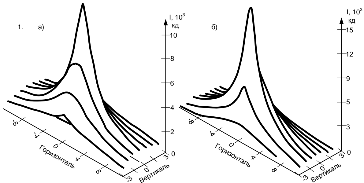
а) ближнє світло фар; б) дальнє світло фар
