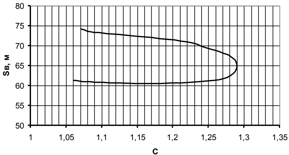
Рис. 6. Залежність дальності видимості S_B від коефіцієнту засліпленості C
