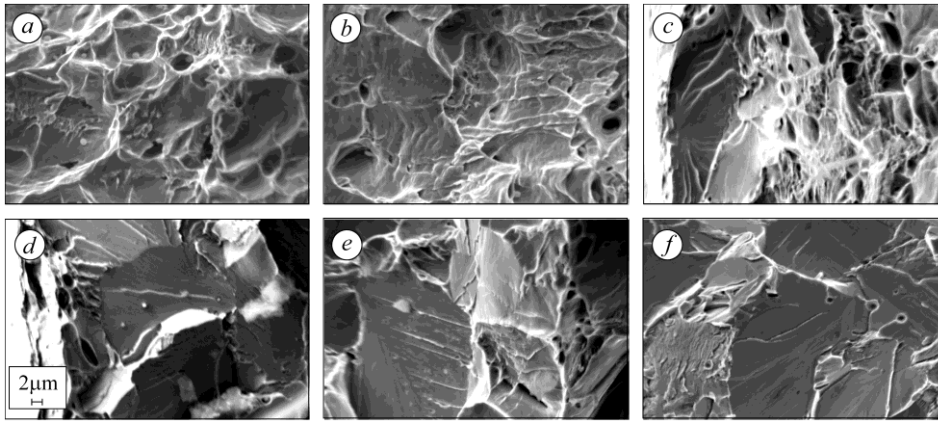
Рис. 2. Фрактографічні особливості руйнування сталі Ст3 у станах № 1 (а, с, е) та № 2 (b, d, f) за випроб на ударну в'язкість KCV за температури +20°C (а, b) та -60°C (с-f) поблизу вершини надрізу (а-d) та на віддалі 5 mm від нього (е, f).
