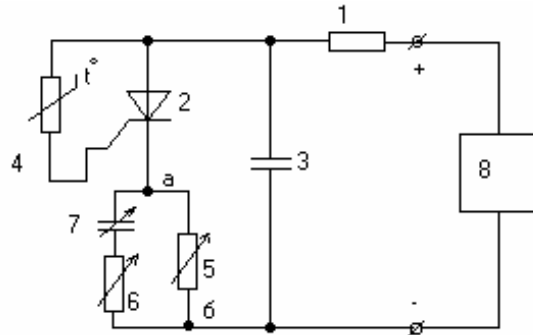
Рисунок 1.7 – Схема перетворювача температури
