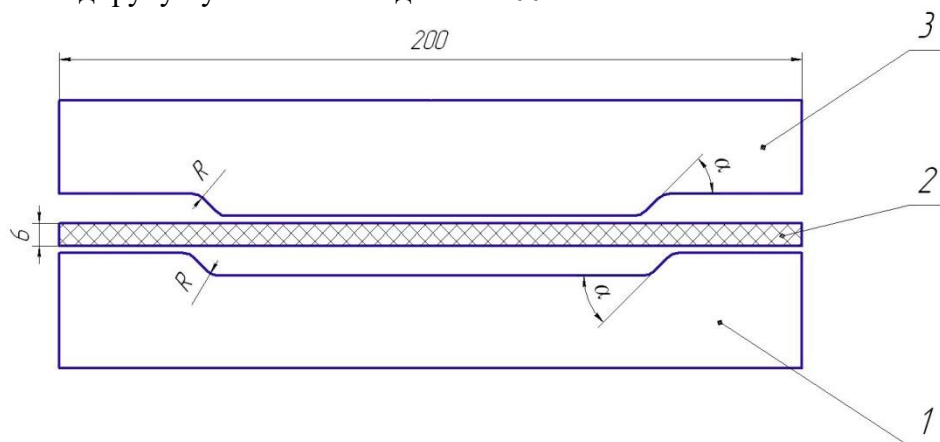
Рис. 1. Геометрична модель:
