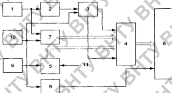
Рис. 3. Функціональна схема бортового вимірювача, яка використовує мікро-ЕОМ з каналом прямого доступу до оперативної пам'яті [8]: 1-контрольний виявлювач сигнальних імпульсів «туди-назад»; 2-порогова схема; 3-пристрій керування обміном; 4-комутатор зовнішніх пристроїв; 5-лічильник числамасштабних імпульсів; 6-генератор масштабних імпульсів; 7-аналого-цифровий перетворювач; 8-мікро-ЕОМ з каналом прямого доступу в пам'ять; 9-лічильник адрес; 10-генератор тактових імпульсів; 11-сигнал опорного часу
