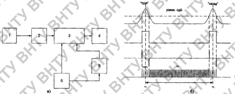
Рис. 2. Рекомендований ІСАО цифровий вимірювач кутових координат [11] а) функціональна схема: 1-контрольний виявлювач кутових сигналів «туди-назад»; 2-порогова схема; 3-комутатор частоти; 4-реверсивний лічильник; 5-подільник частоти на 2; 6-генератор масштабних імпульсів; б) часові діаграми роботи
