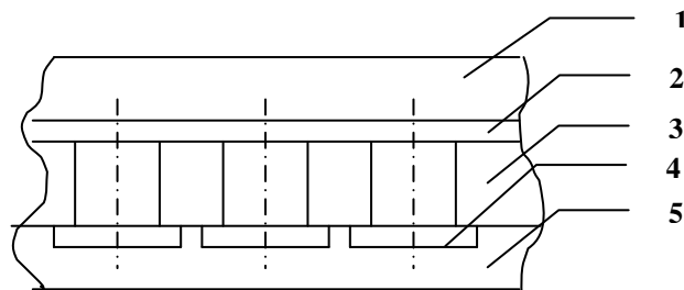
Рис. 5.5. Газорозрядна панель постійного струму
