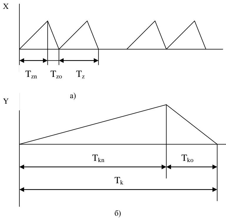
Рис. 5.2. Часові діаграми рядкової X та кадрової Y розгортки
