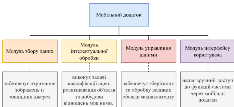
Рис. 1. Компоненти архітектури програмної системи
