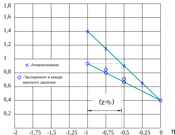
Рис.1. Диаграмма пластичности стали Р 9, построенная в условиях наложения гидростатического давления \varepsilon_p(\eta_2) и без давления \varepsilon_p(\eta_1)
