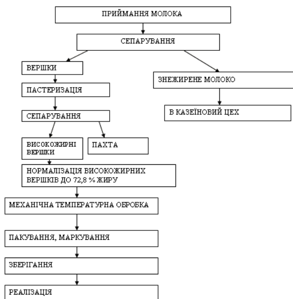
Рис. 2. Загальна технологічна схема
