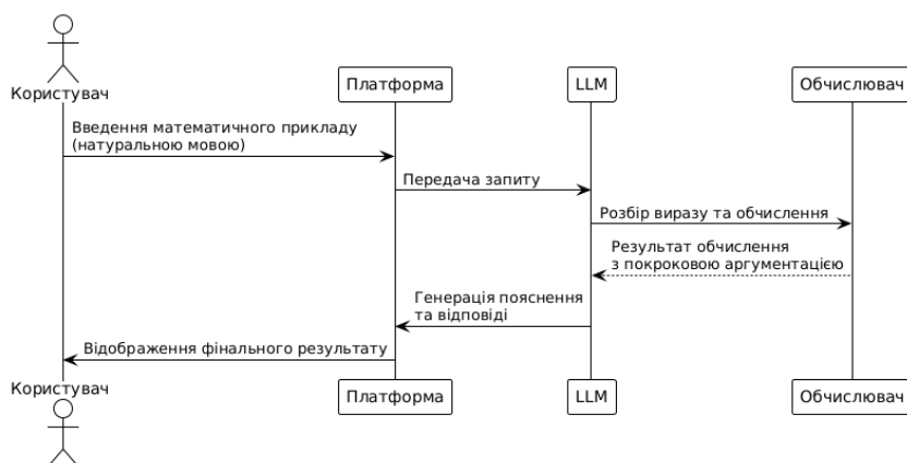
Рис. 1. UML-діаграма послідовностей інтеграції дистильованої великої мовної моделі (LLM) для автоматичного обчислення математичних завдань
