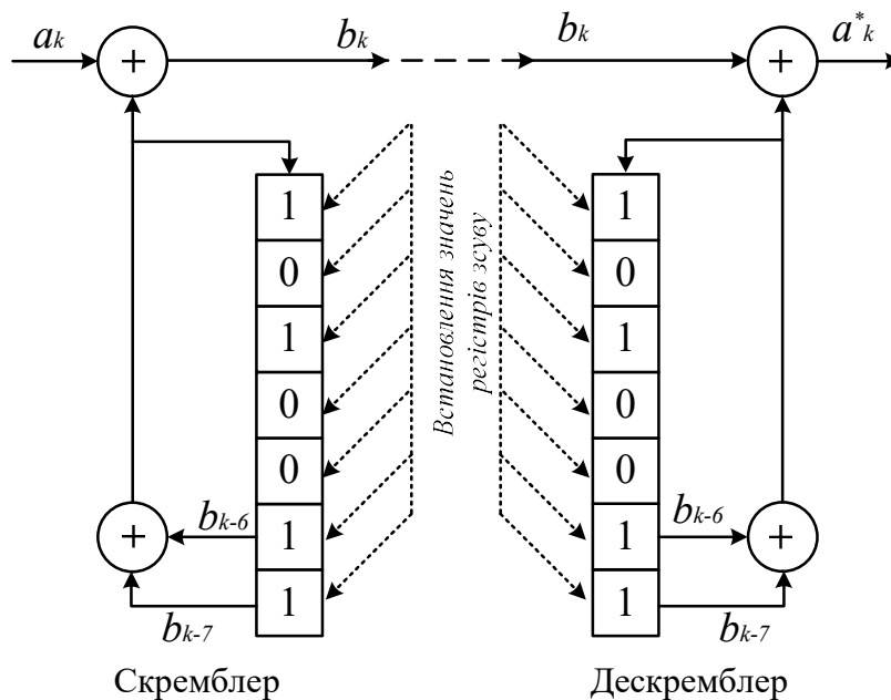
Рисунок. 5.6 – Адитивні скремблер і дескремблер.
