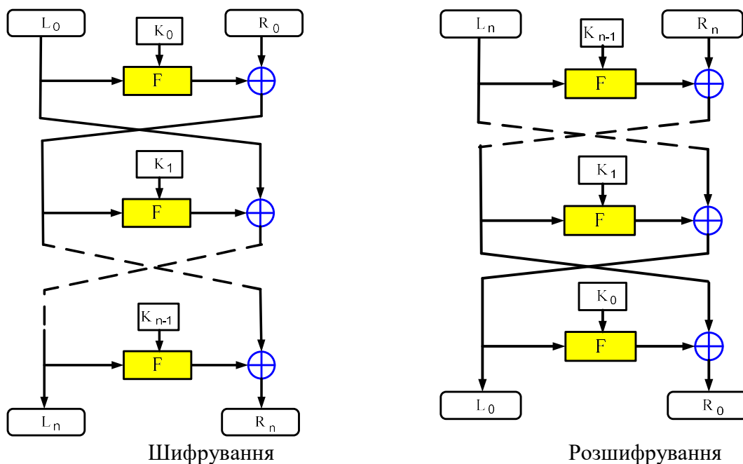
Рисунок 6.3 – Мережа Фейстеля
