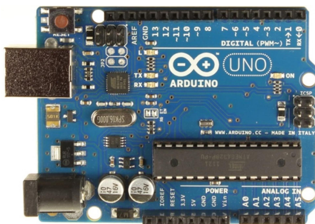
Рисунок 1.6 – Зовнішній вигляд Arduino Uno R3
