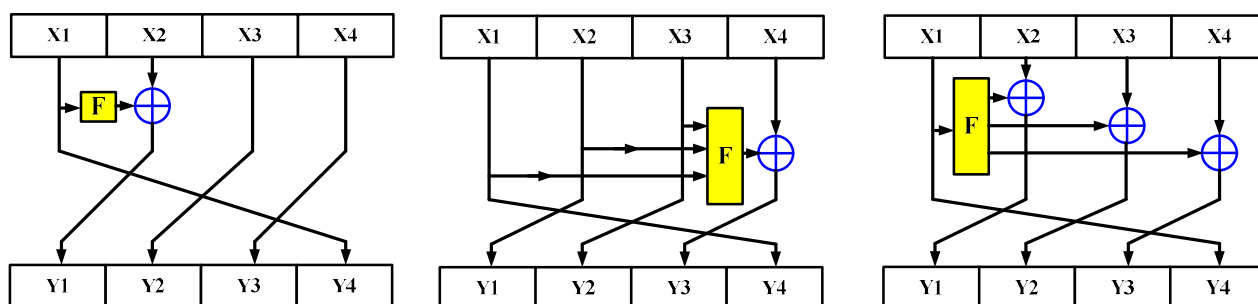
Рисунок 6.4 – Модифікована мережа Фейстеля
