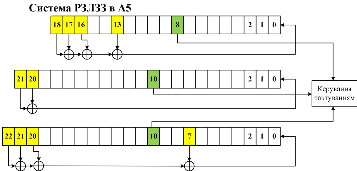
Рисунок 5.4 – Система реєстрів в алгоритмі A5/1
