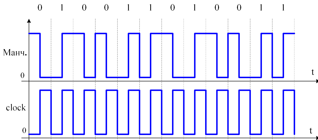
Рисунок 3.4 – Манчестерське кодування
