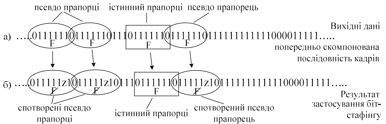
Рисунок 2.2 – Використання біт-стафіngu
