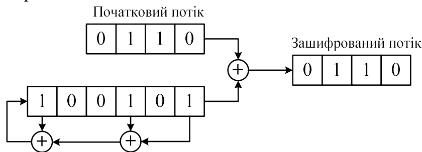
Рисунок 5.7 – Структура шести розрядного скремблера
